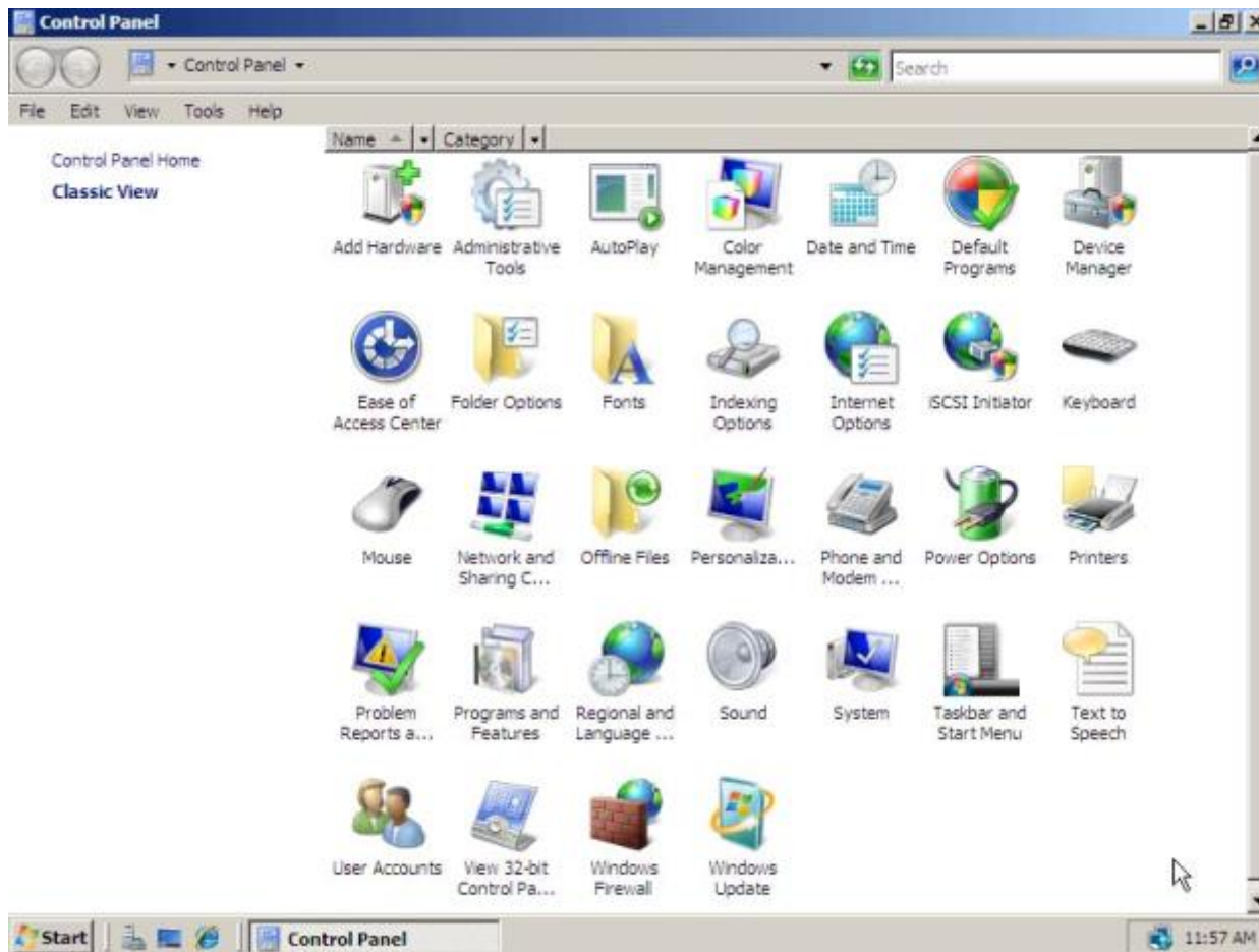
Рис. 35.5. Панель управления
