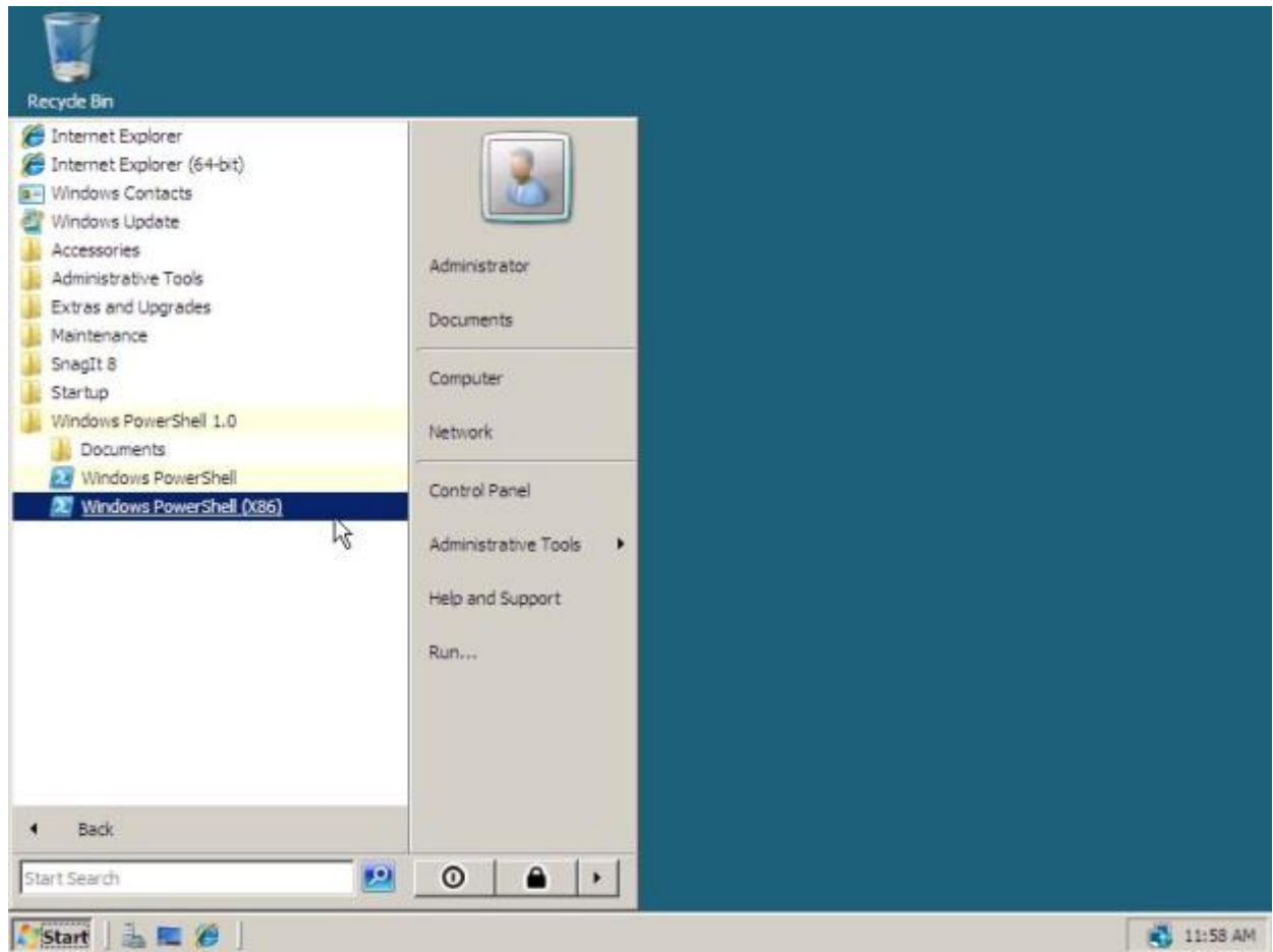
Рис. 35.16. Запуск PowerShell
