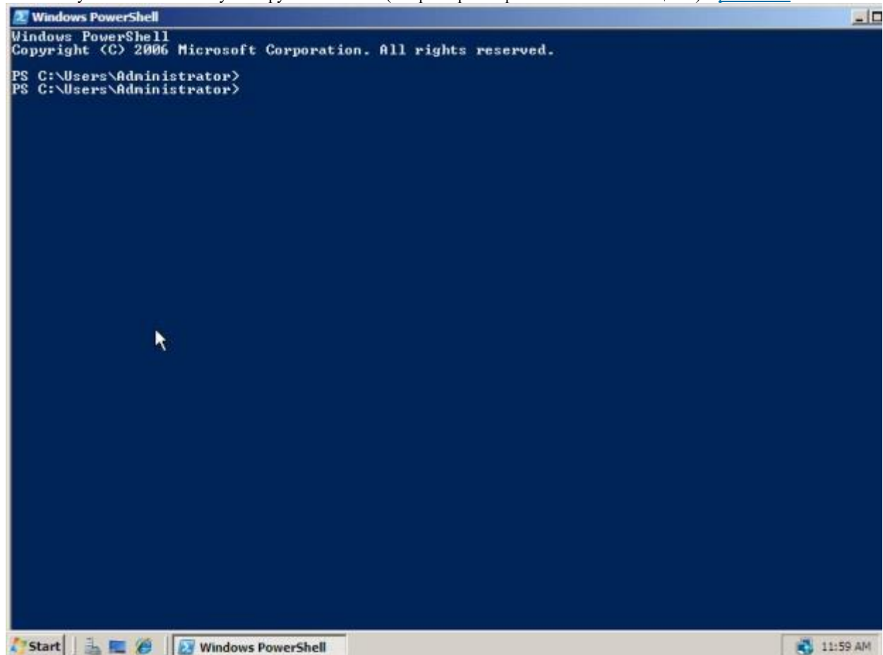
Рис. 35.16. Запуск PowerShell
